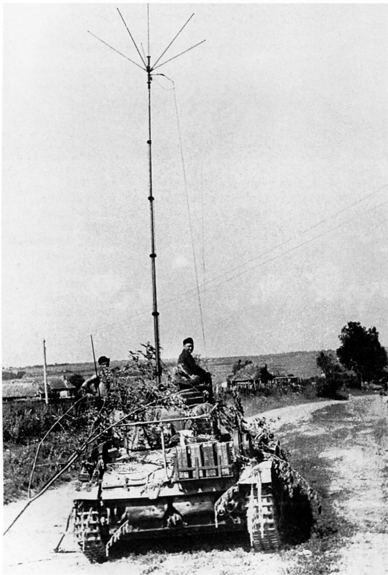
Командирский танк Pz.Bf. Wg III Ausf. E с развернутой антенной. Группа армий «Юг», май 1942 года (РГАКФД).
