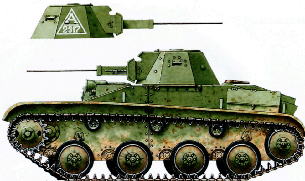
Танк Т-60 предположительно из состава 121-й танковой бригады. Южный фронт, май 1942 года. Оознавательные знаки нанесены только на правой стороне башни.
