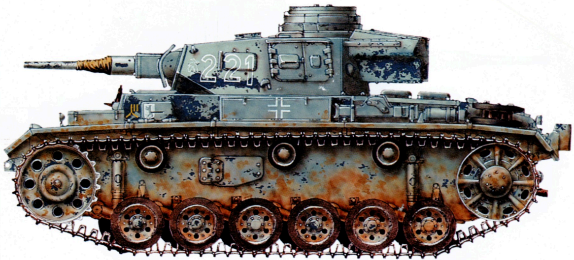
Танк Pz.III G3-й танковой дивизии вермахта. Юго-Западный фронт, март 1942 года. Поверх первоначального темно-серого цвета перекрашен более светлой серой краской.
